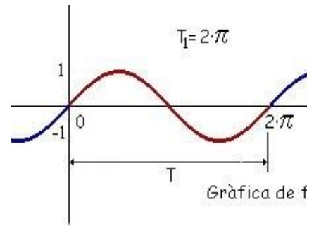
Periodo de las ondas sonoras con la función seno.
