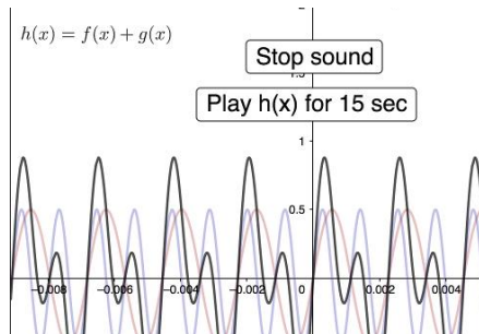
Amplitud de la función seno en la gráfica de ondas sonoras.
